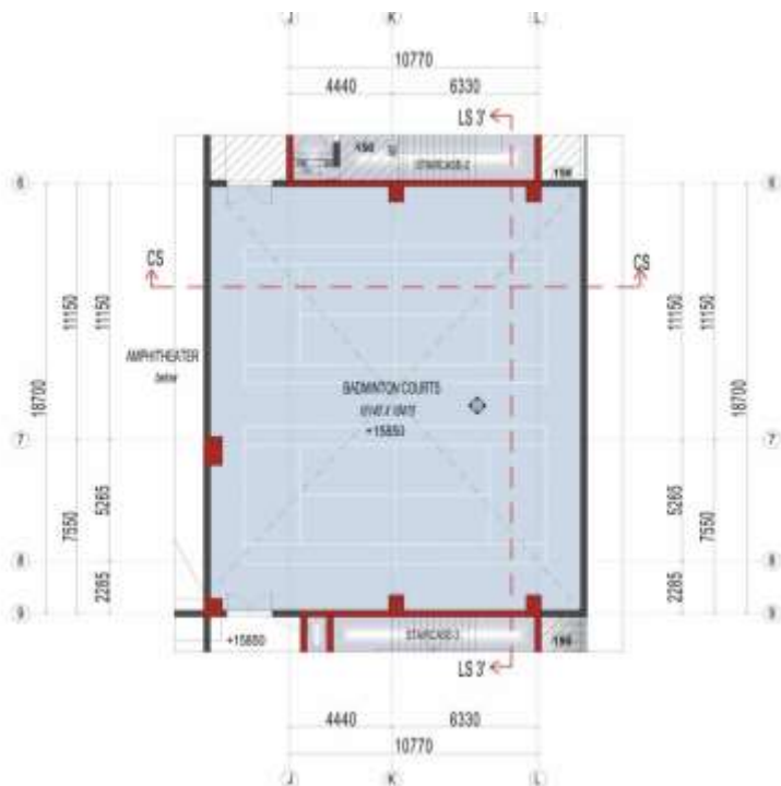
BADMINTON COURT -PART PLAN
